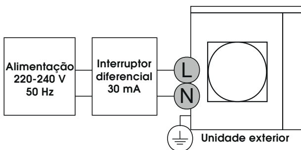
Unidade exterior monofásica
